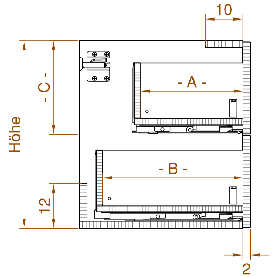
Schnitt B-B
