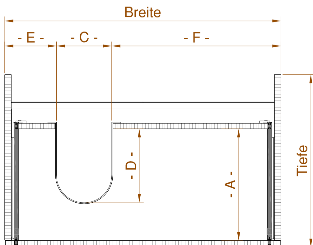
Schnitt A-A mit Siphonausschnitt Position frei wählbar (für die obere Schublade optional auswählbar)
