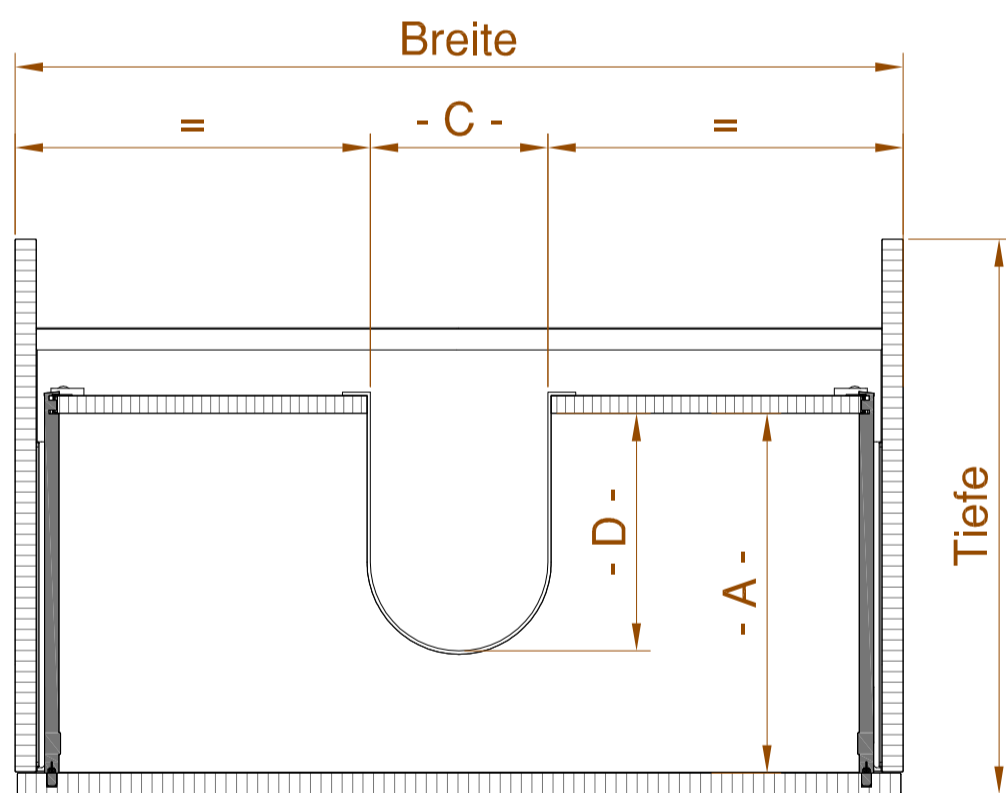
Schnitt A-A mit Siphonausschnitt in der Mitte (für die obere Schublade optional auswählbar)
