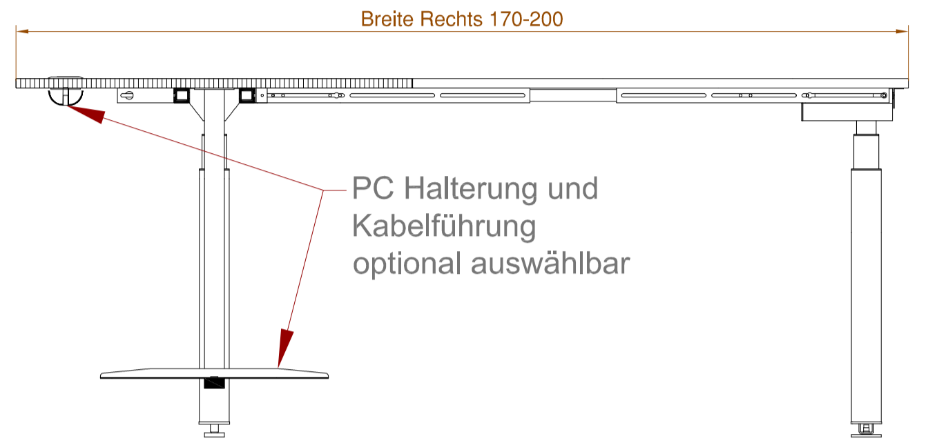
Schnitt A-A
