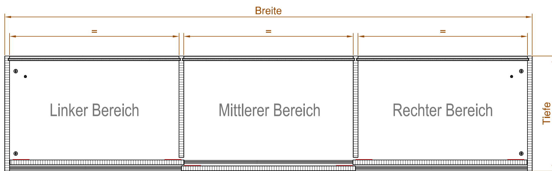
Schnitt A-A
