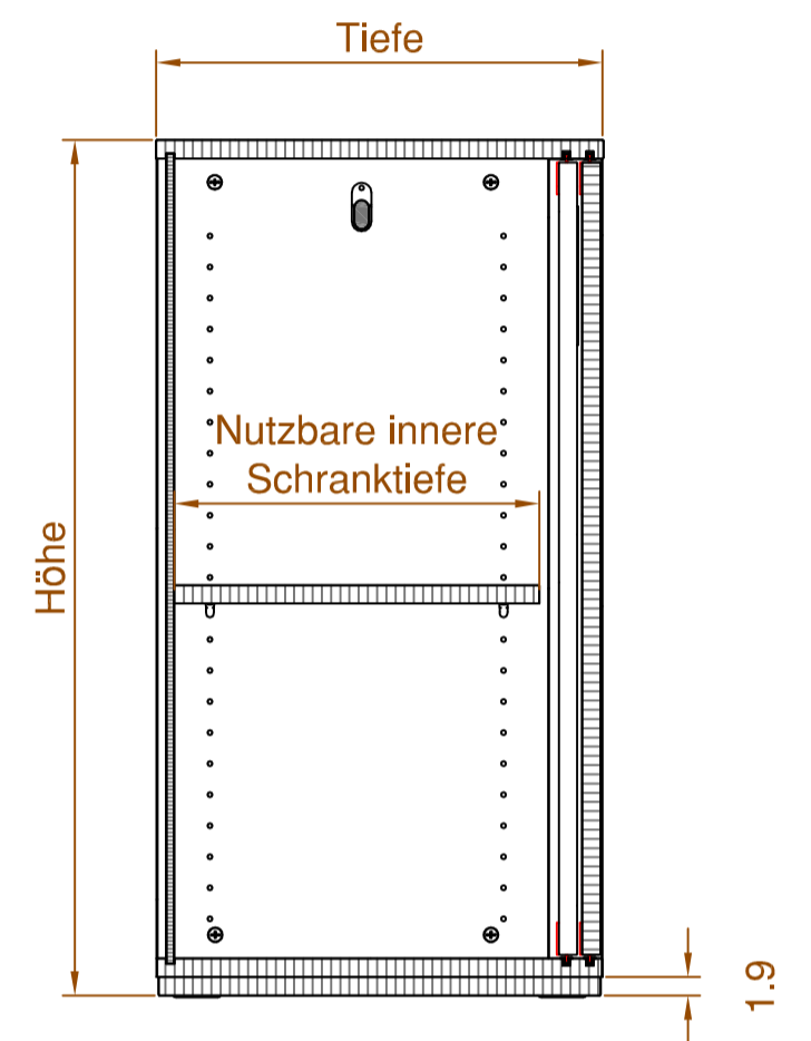
Schnitt B-B
