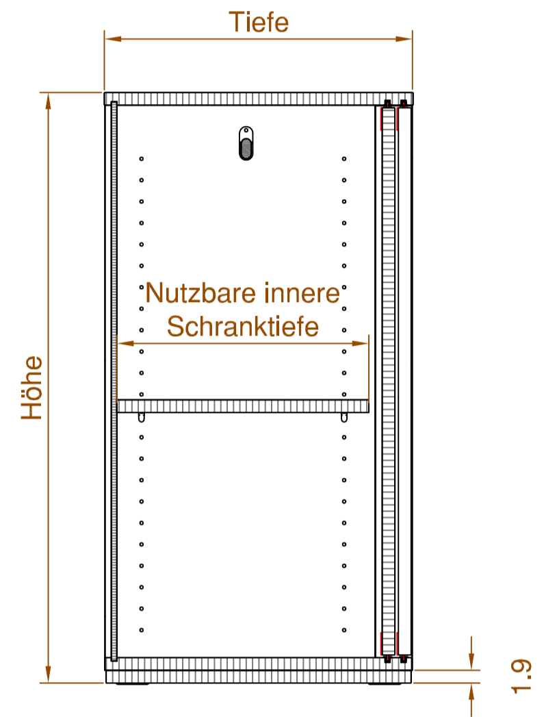
Schnitt B-B
